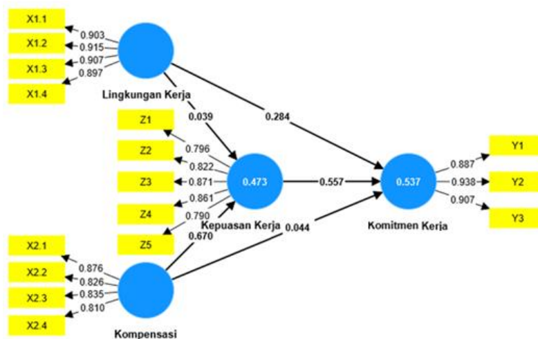
Gambar 1 Algoritem
