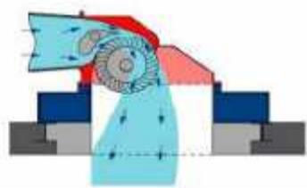
Gambar 3. Turbin Cros Flow (Sumber : Haimerl, L.A., 1960)
