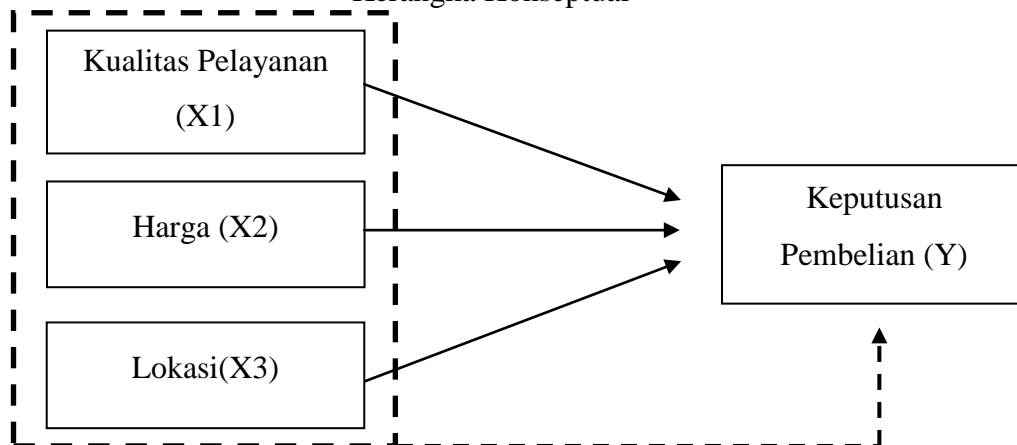
Gambar 1 Kerangka Konseptual
