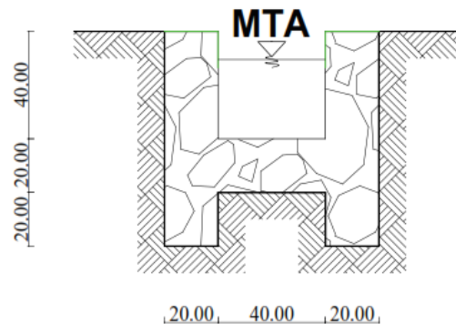
Gambar 9. Konstruksi Saluran Trapesium Saluran
