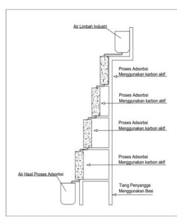
Gambar 4. Desain Rencana Sumber : Penulis, 2024.
