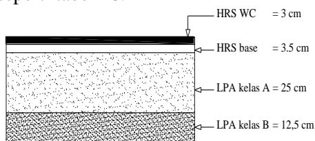
Gambar 11. Struktur Perkerasan
