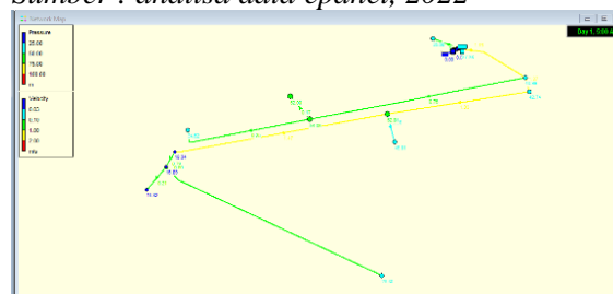
Gambar 7. Analisa Jaringan Epanet Sumber : analisa data epanet, 2022
