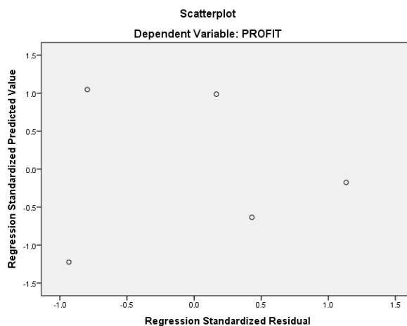
Gambar 3. Kehomogenan Data
