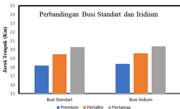
Gambar 6. Perbandingan Jarak tempuh Busi Standar dan Busi Iridium
