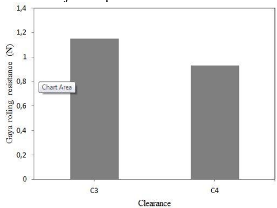
Grafik 7. Rolling resistance C3 dan C4
