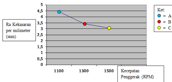
Gambar 12. Grafik Rata-Rata Tingkat Kekasaran Benda Kerja
