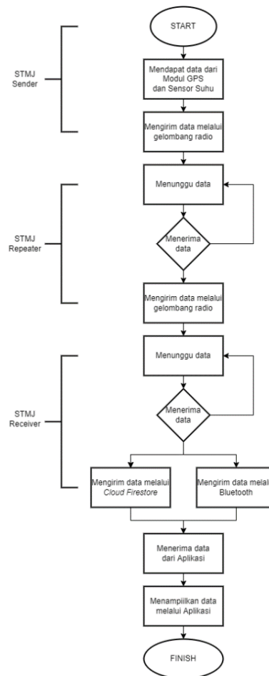
Gambar 13. Flowchart perancangan sistem
