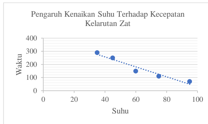
Gambar 4. Grafik pengaruh kenaikan suhu terhadap kecepatan kelarutan zat
