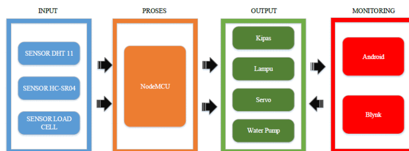
Gambar 1. Blok diagram sistem smart cage
