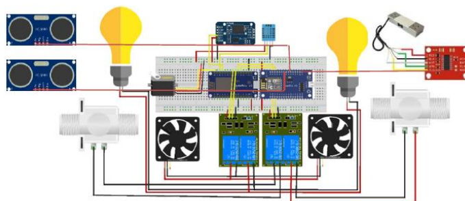
Gambar 2. Rancangan rangkaian elektronika pada smart cage
