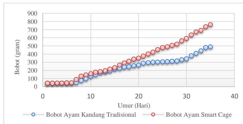
Gambar 9. Perbandingan Bobot Ayam Pada Smart Cage dengan Bobot Ayam Pada Kandang Konvensional
