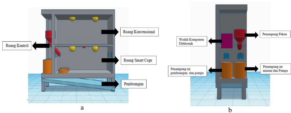
Gambar 3. Desain (a) bagian-bagian kandang (b) ruang kontrol
