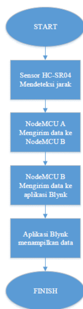
Gambar 7. Flowchart kapasitas pakan dan minum
