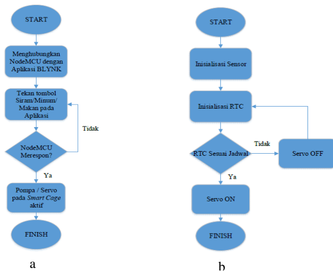
Gambar 6. Flowchart sistem kontrol pemberi pakan, minum, dan pembersih kandang (a) menggunakan smartphone android (b) secara otomatis
